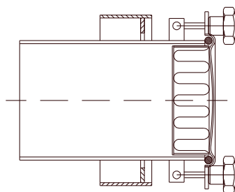
Draufsicht
